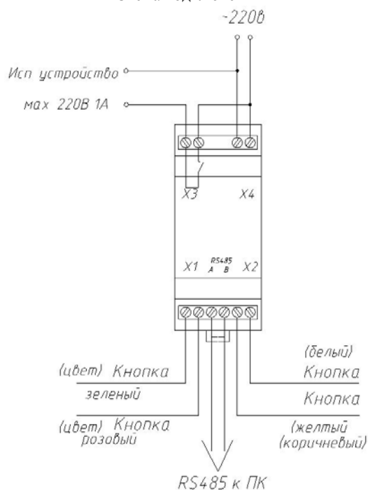
Схема подключения
